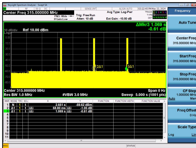
315 MHz: Burst 1
