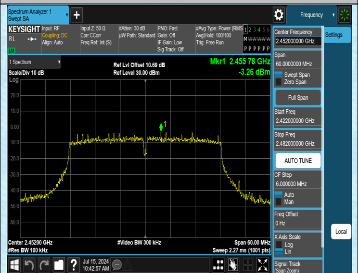
11N40ISO-Ant1-2452-0-Reference-PASS
