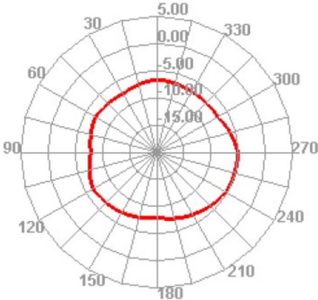
2400.000MHz H
