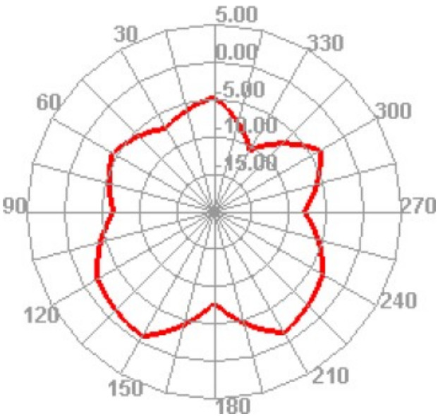
2400.000MHz E1
