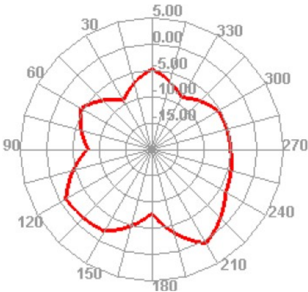
2400.000MHz E2
