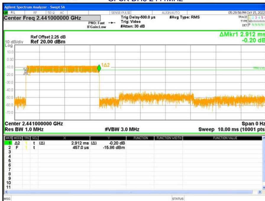
GFSK DH5 2441MHz
