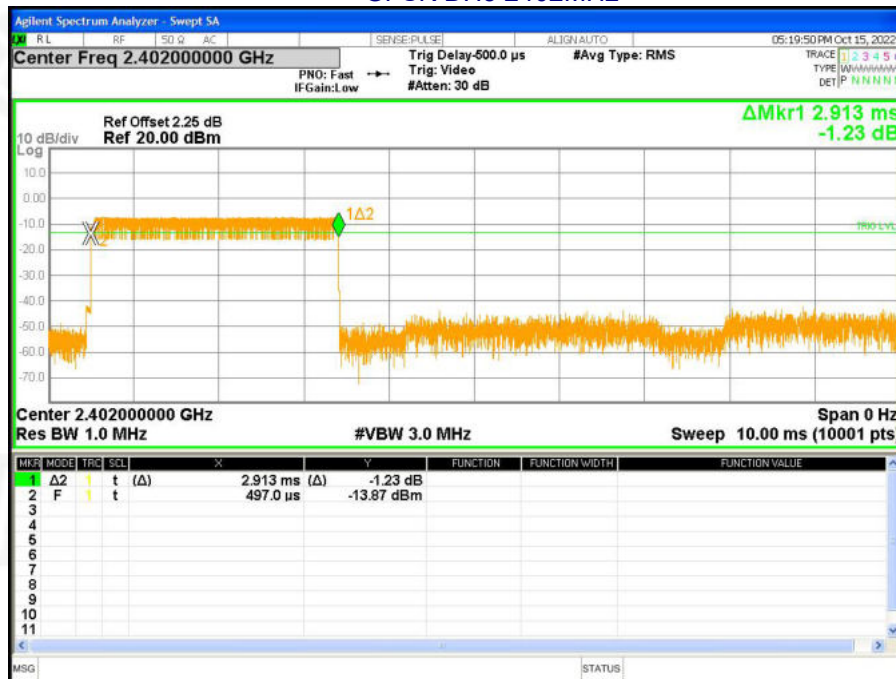
GFSK DH5 2402MHz
