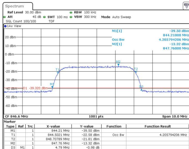
Band5-4233-2-4.78
