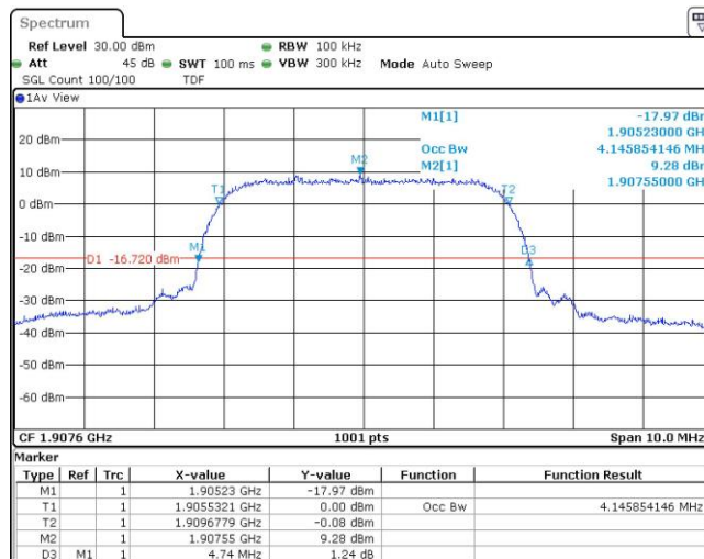
Band2-9538-3-4.74
