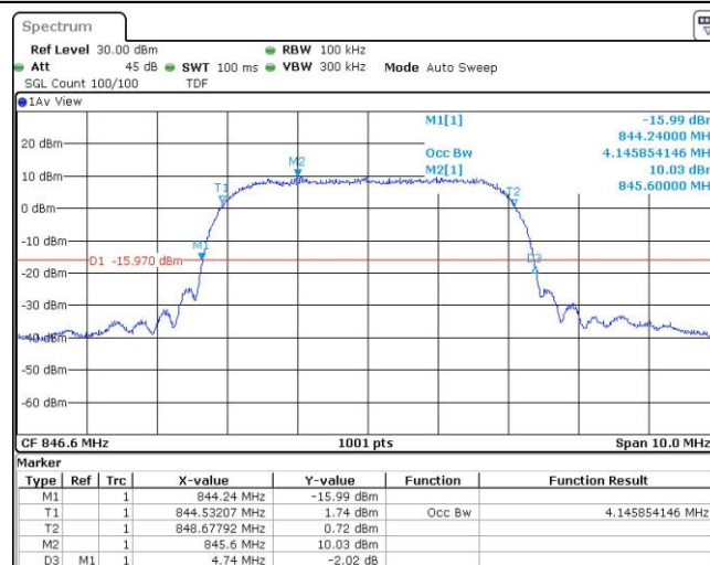
Band5-4233-2-4.73
