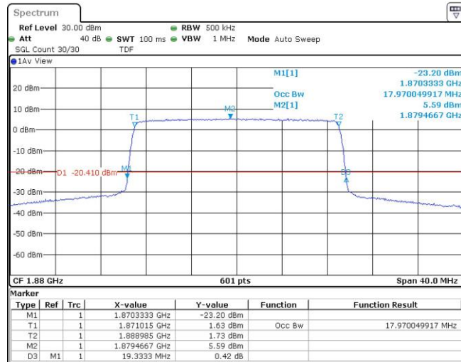
Band2-20MHz-QPSK-19100-1RB#99
