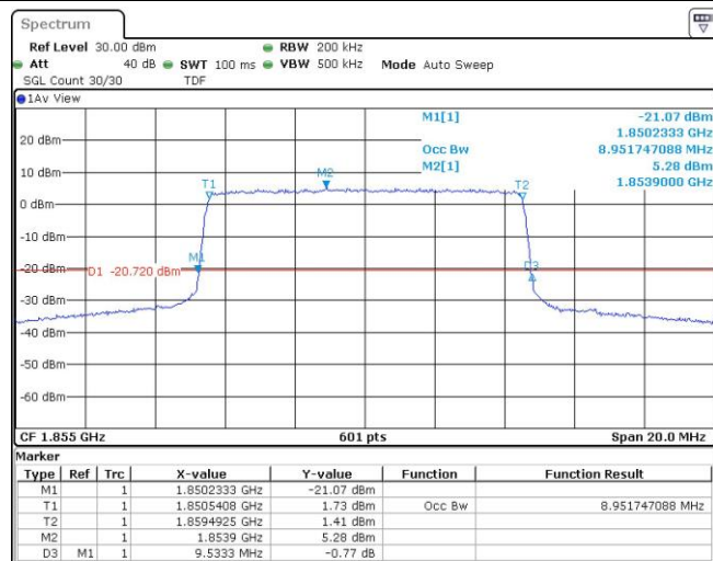
Band2-10MHz-QPSK-18650-50RB#0
