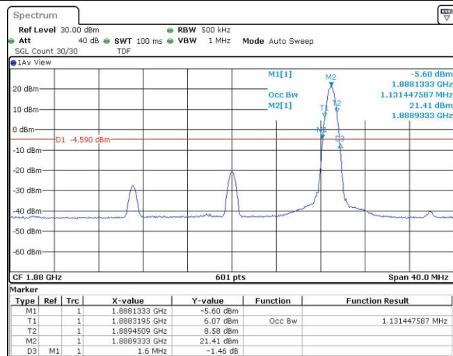
Band2-20MHz-16QAM-18900-1RB#99
