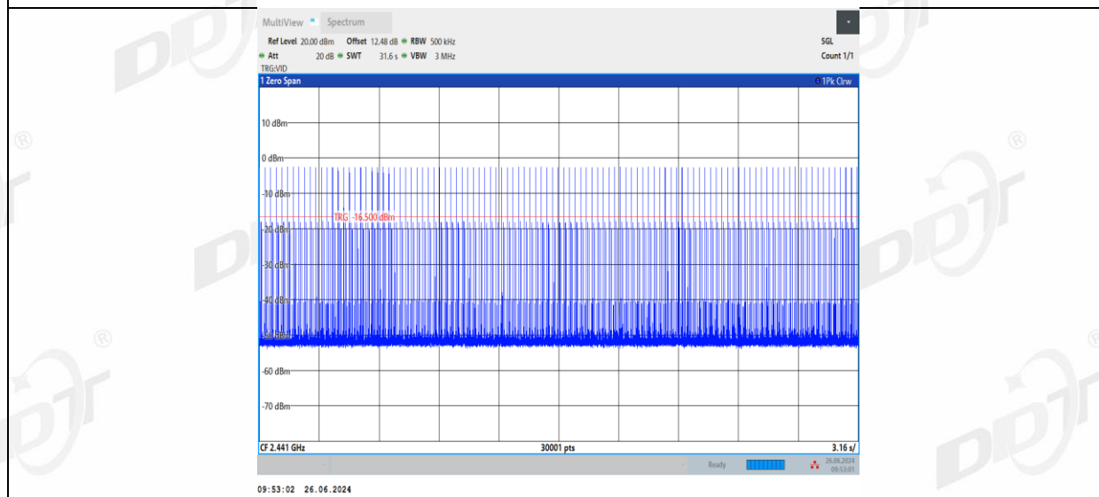
3DH3_Left side_Hop
