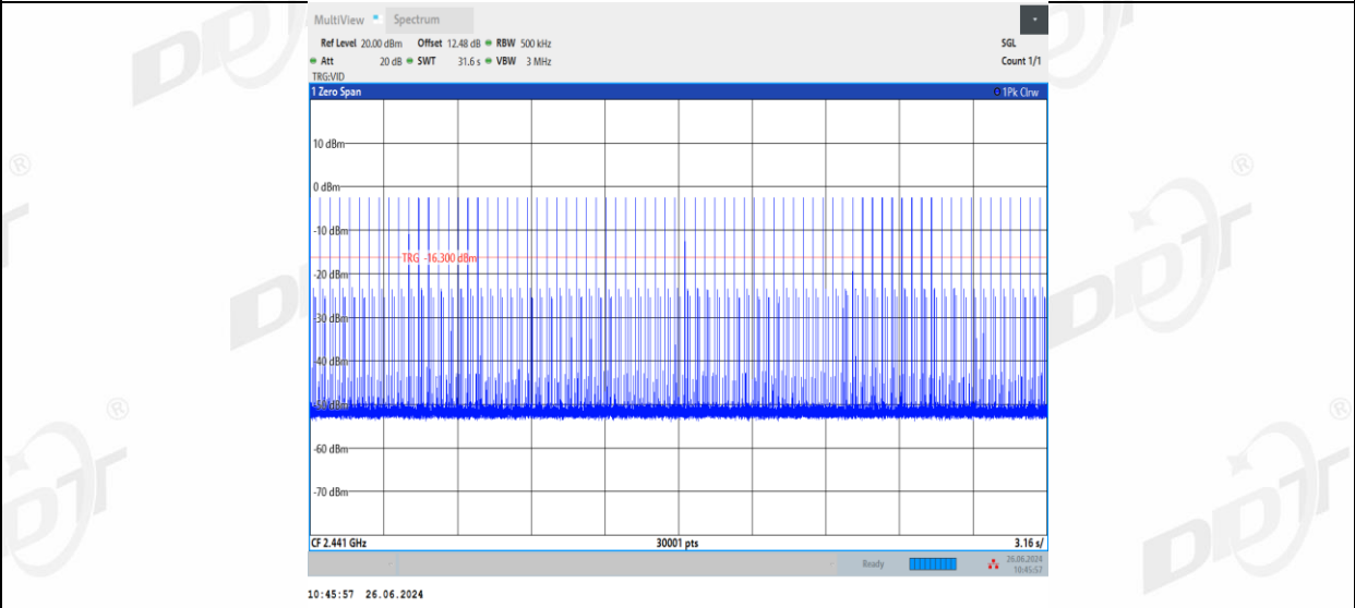
2DH1_Right side_Hop
