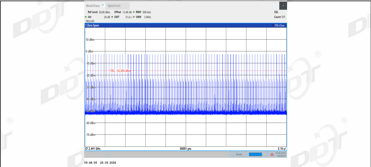
DH5_Left side_Hop
