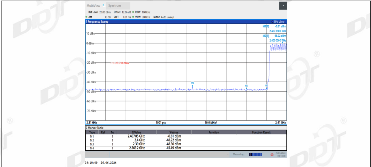
2DH5_Left side_Low_Hop_2402
