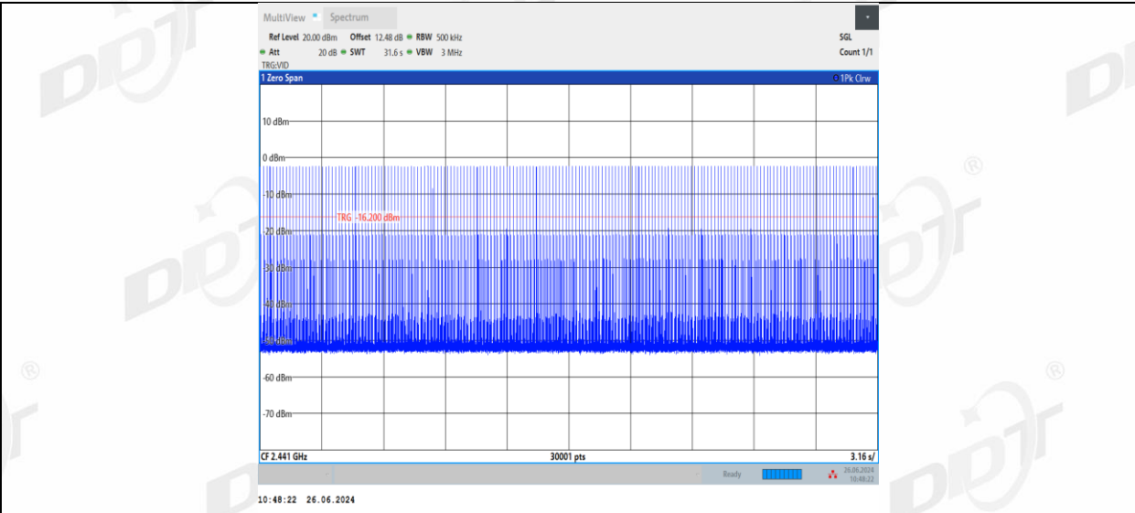
DH3_Right side_Hop
