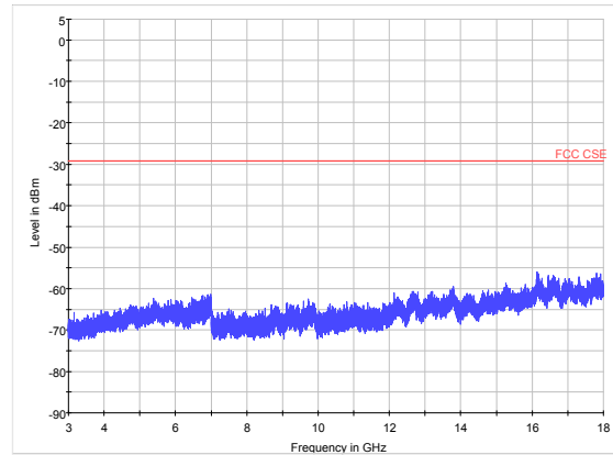
802.11n (HT20) CH6 3GHz to 18GHz
