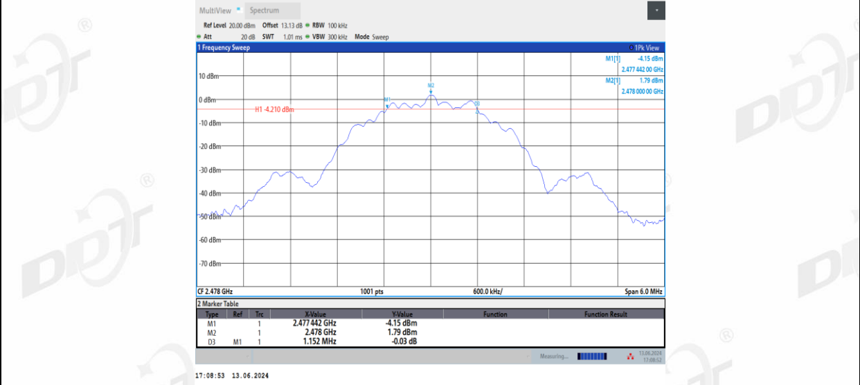
BLE_2M_Right side_2478
