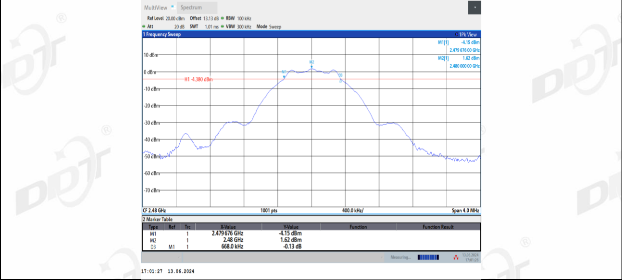
BLE_1M_Right side_2480
