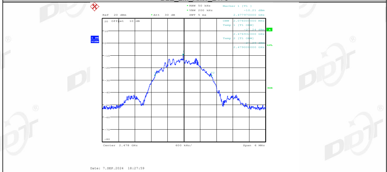
BLE_2M_Ant1_2478
