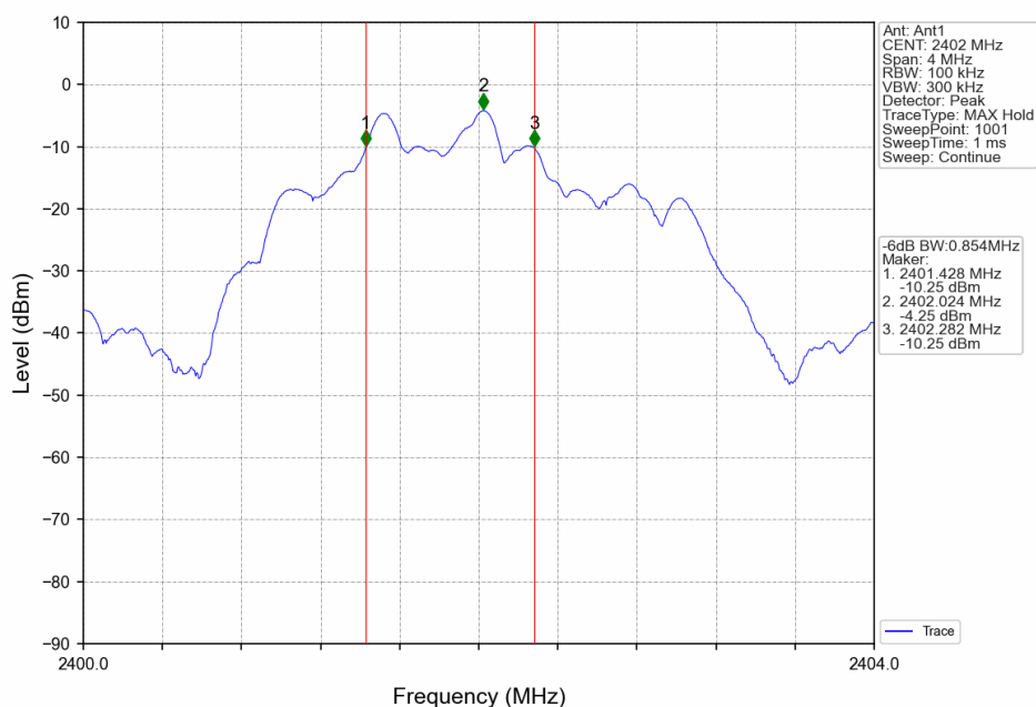
GFSK 2M LCH 240GFSK 2MHz Ant1 NTN
