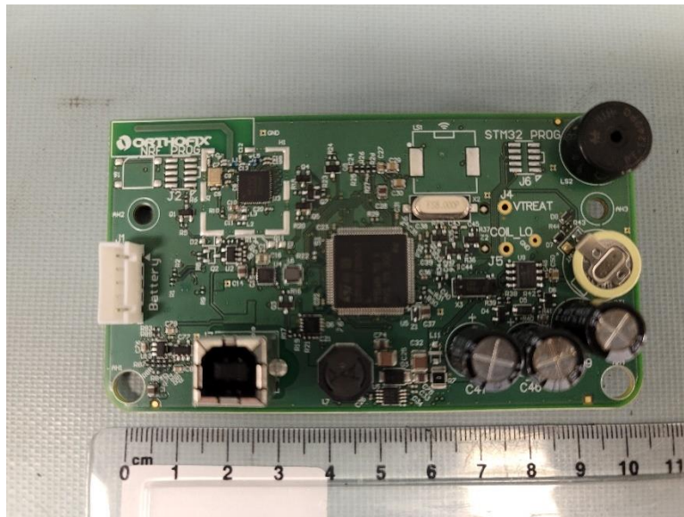
Figure 54 - 5314LCM PCA Top
