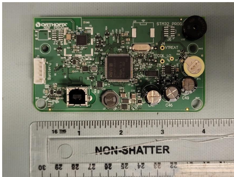
Figure 6 - 5212CM PCA Top
