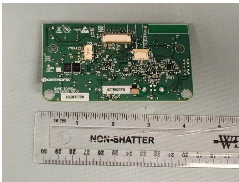
Figure 7 - 5212CM PCA Bottom
