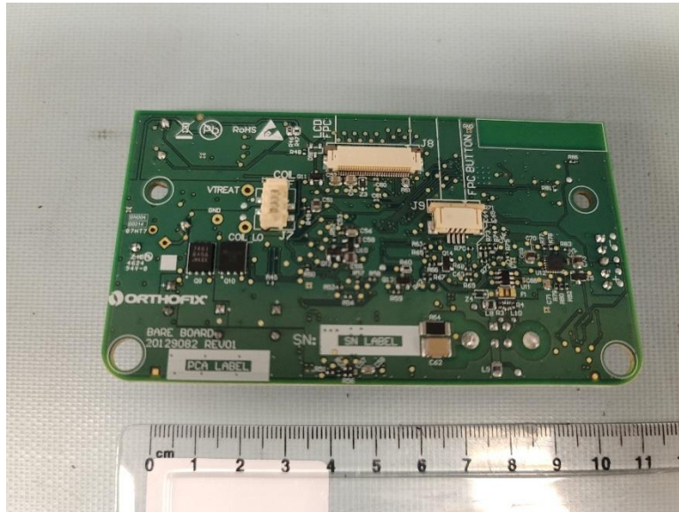
Figure 55 - 5314LCM PCA Bottom
