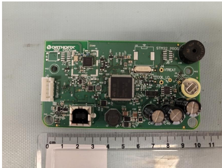
Figure 38 - 5313CM PCA Top
