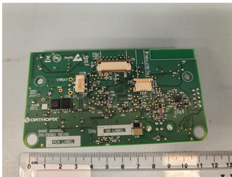
Figure 31 - 5303CM PCA Bottom
