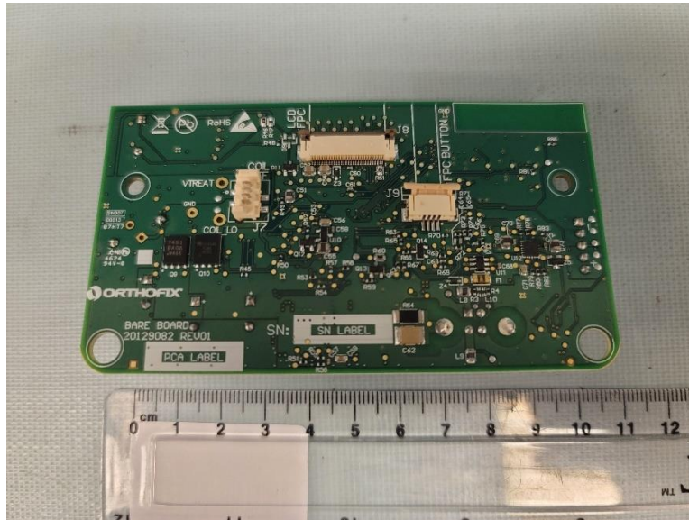
Figure 39 - 5313CM PCA Bottom
