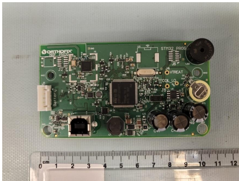
Figure 30 - 5303CM PCA Top
