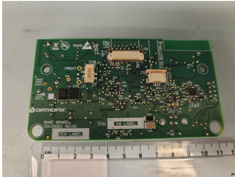
Figure 63 - 5315CM PCA Bottom
