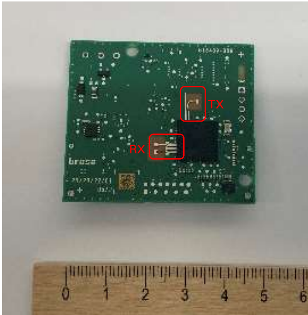
R-HFA PCBA Top Side
