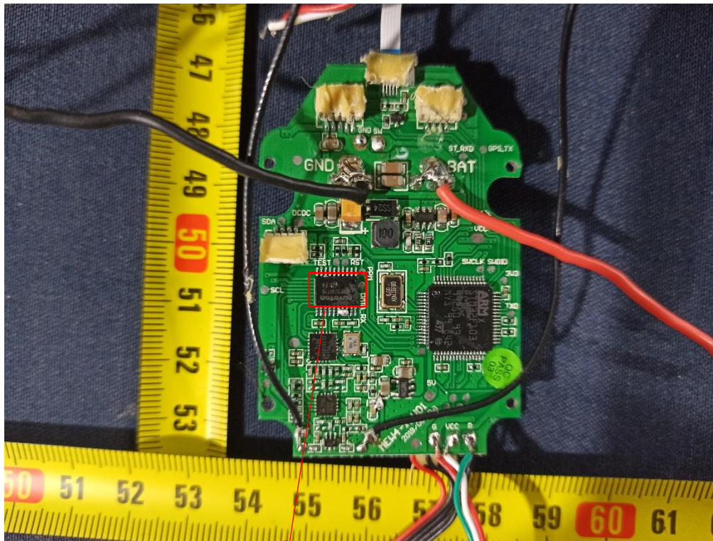
2.4G Module: N76E003AT20
