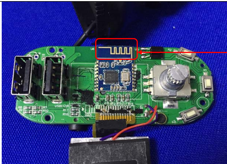
Antenna
