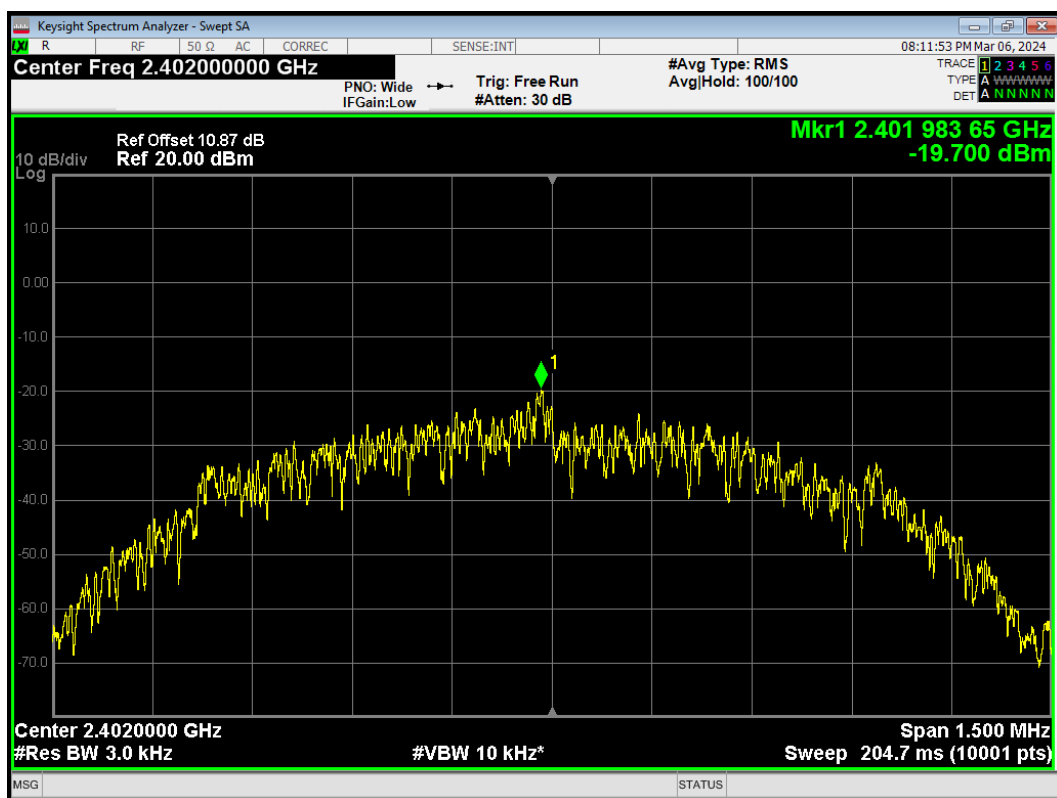
PSD BLE 2402MHz
