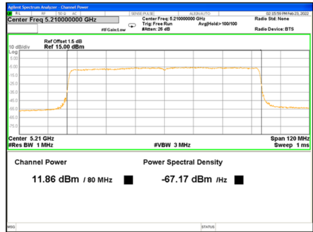
5210MHz_ax80_Ant A
