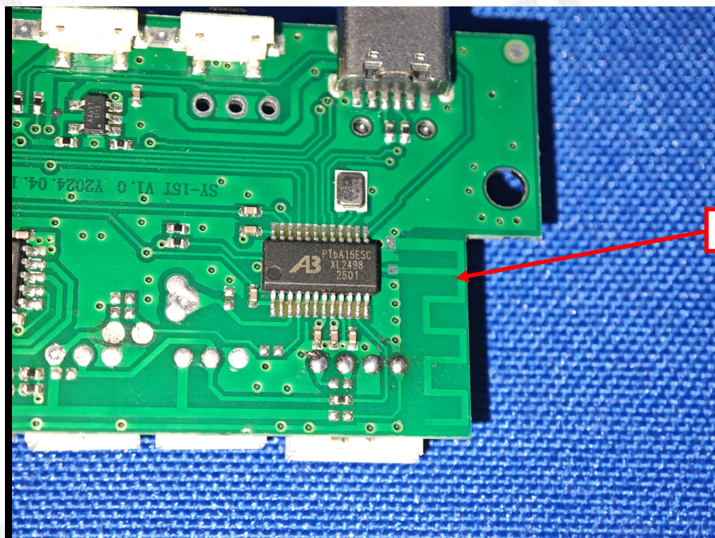
BLE Antenna
