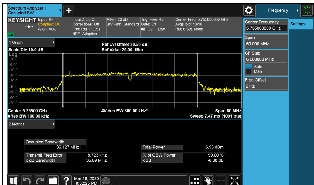
802.11n-HT40-5755MHz
