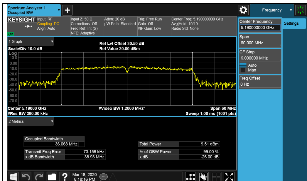
802.11n-HT40-5190MHz
