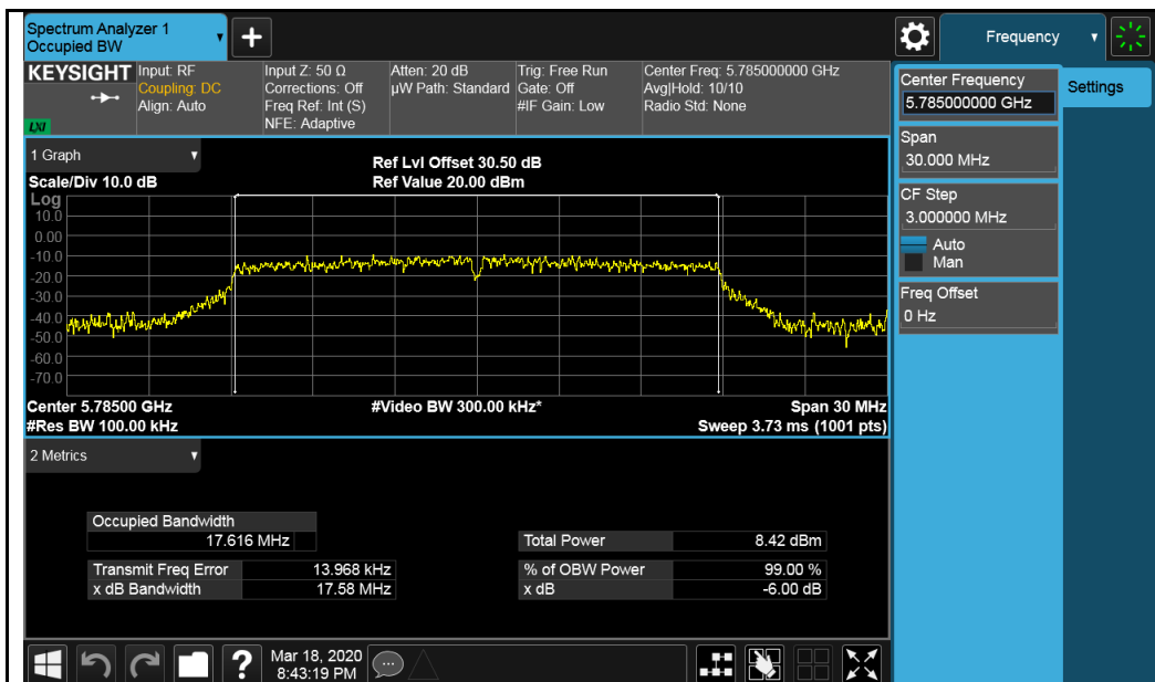
802.11n-HT20-5785MHz
