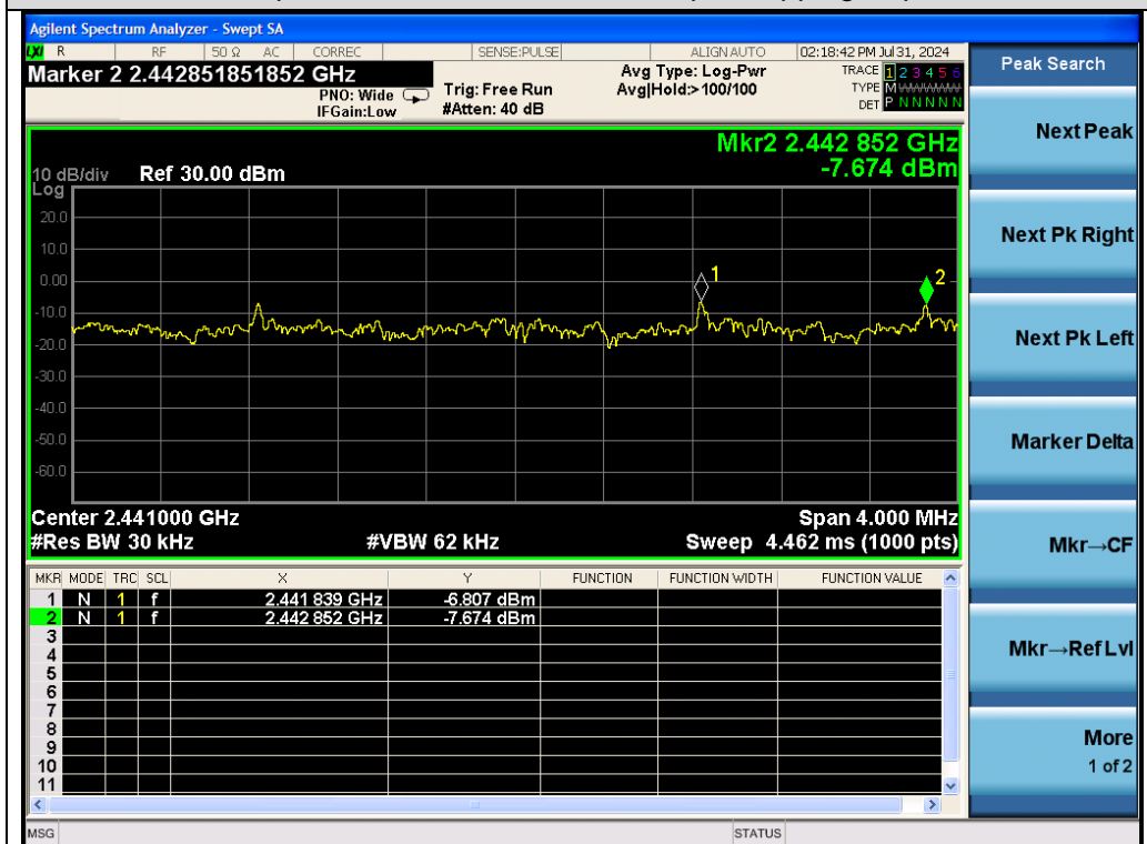
Test_Graph_EDR_HOP_ANT1_NA_3Mbps_Hopping Separation
