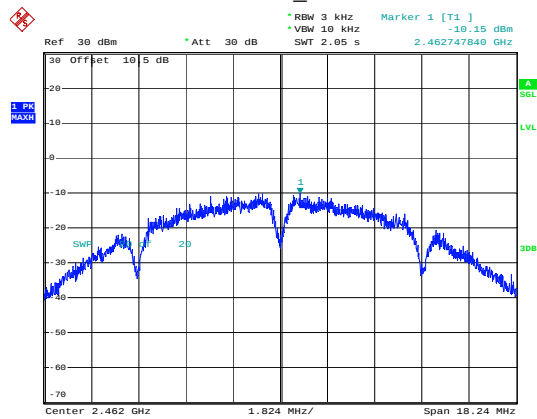
802.11b_2462MHz
