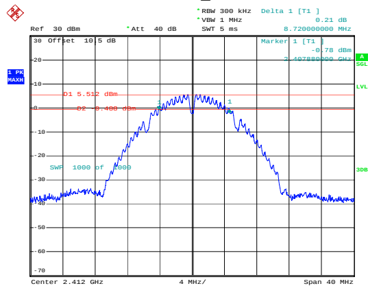
802.11b_2412MHz
