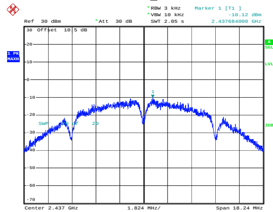
802.11b_2437MHz
