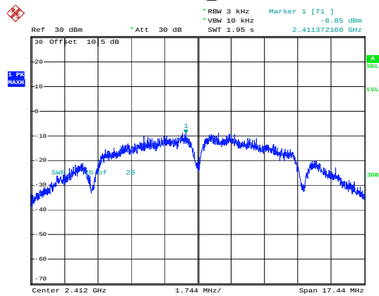
802.11b_2412MHz
