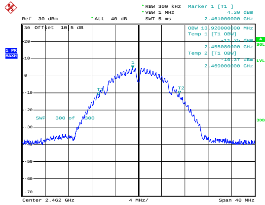
802.11b_2462MHz
