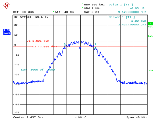
802.11b_2437MHz
