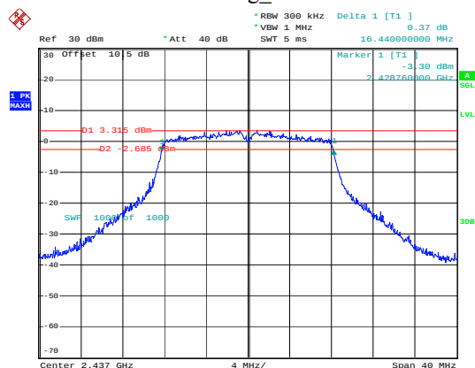
802.11g_2437MHz
