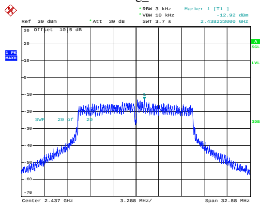
802.11g_2437MHz
