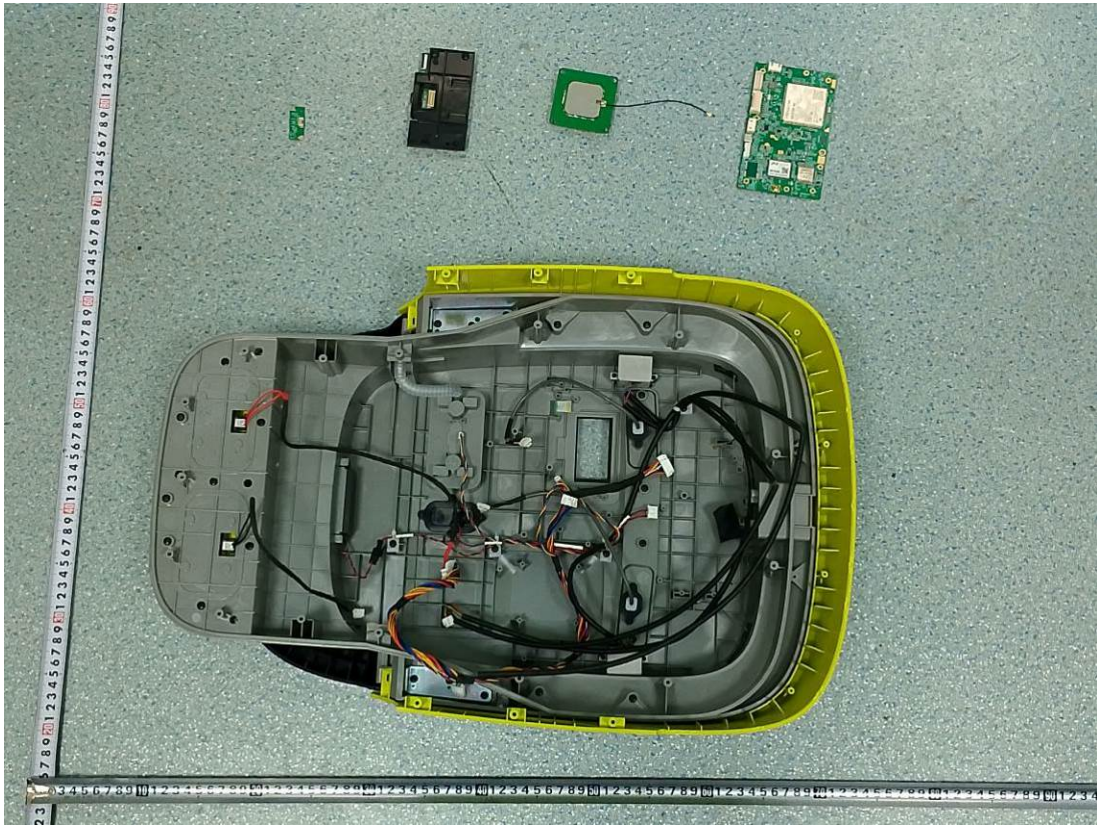
BLE&Wifi Antenna
