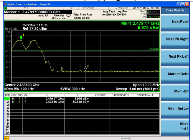
CH78 (Hopping on)
