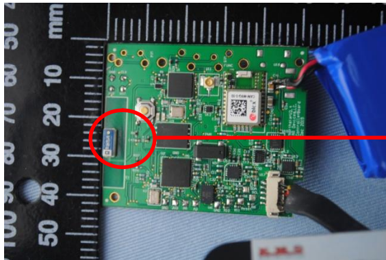
ANT0 TX0/RX0
