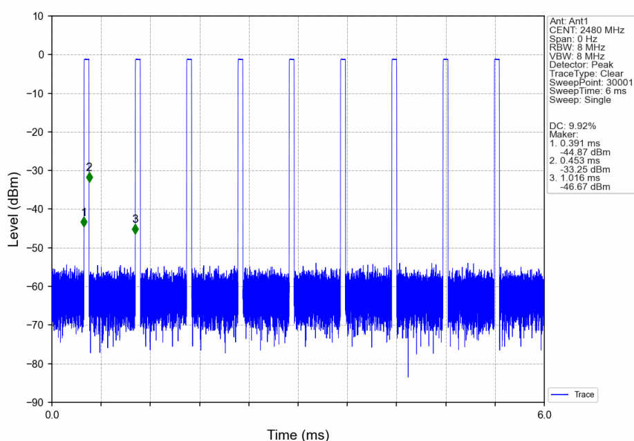
GFSK-2M_HCH_2480MHz_Ant1_NTNV
