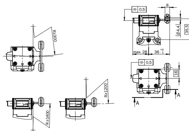
Figure 50: Min. door radii for TR110-XABT angled actuator (mm)
