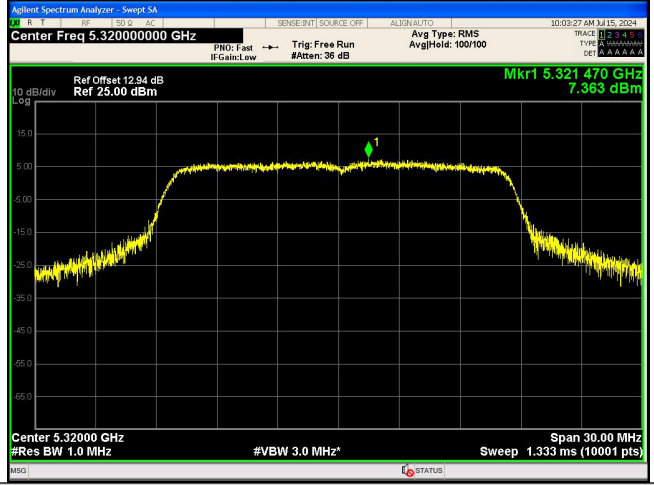
IEEE 802.11a_Channel 64_20MHz_Antenna 0
