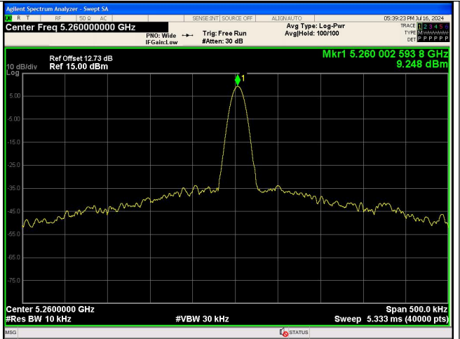
NT/NV_Antenna 0 IEEE 802.11ac_Channel 52_20MHz
