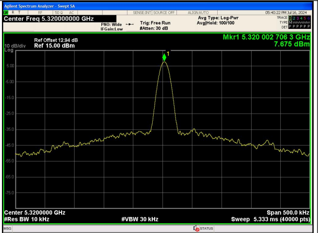
NT/NV_Antenna 0 IEEE 802.11ac_Channel 64_20MHz
