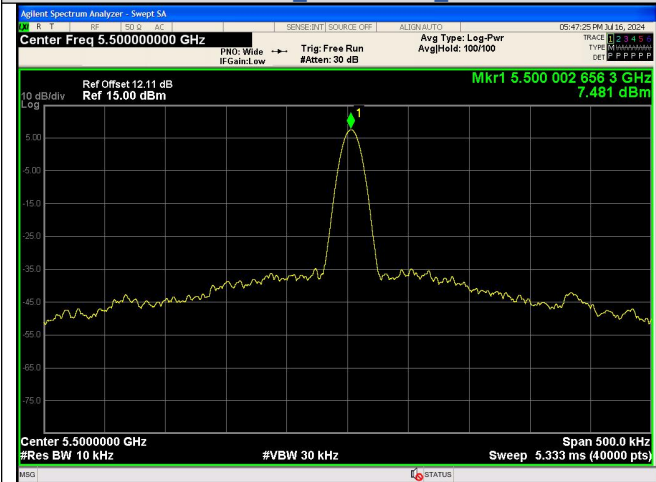
NT/NV_Antenna 0 IEEE 802.11n_Channel 100_20MHz
