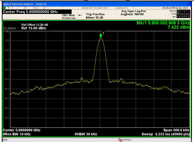
NT/NV_Antenna 0 IEEE 802.11n_Channel 120_20MHz
