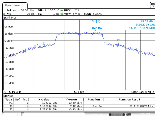
n40_5190MHz_Chain 0
