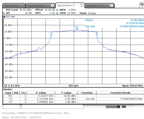
ac80_5210MHz_Chain 0
