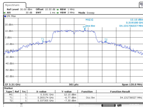
n40_5310MHz_Chain 0
