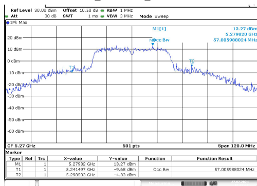
n40_5270MHz_Chain 0
