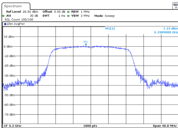
ac20_5200MHz_Chain 0z
