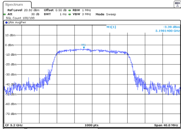
a_5200MHz_Chain 0
