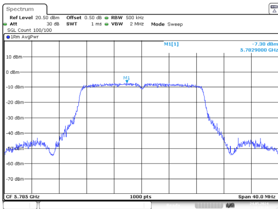
ac20_5785MHz_Chain 0
