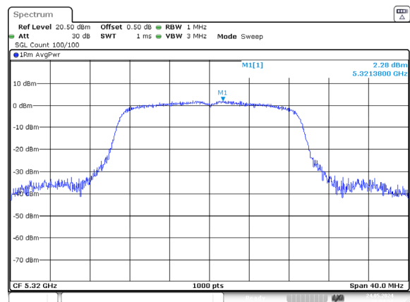
ac20_5320MHz_Chain 0
