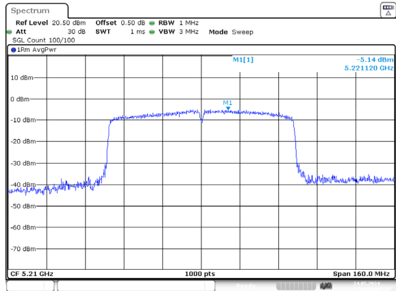
ac80_5210MHz_Chain 0
