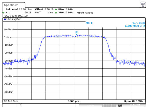
ac20_5500MHz_Chain 0
