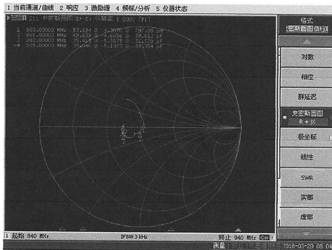
天线阻抗图 4-2
