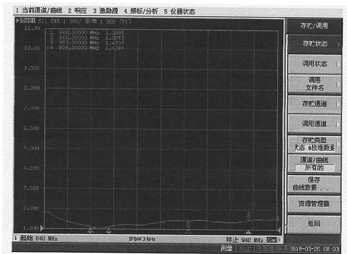
天线阻抗图 4-2
