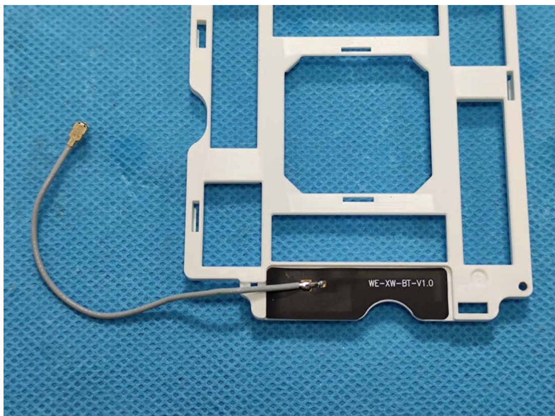
BLE Antenna
