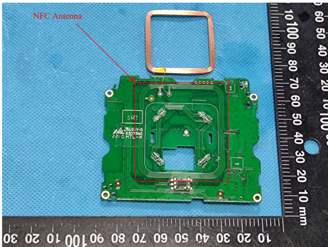
RFID Antenna
