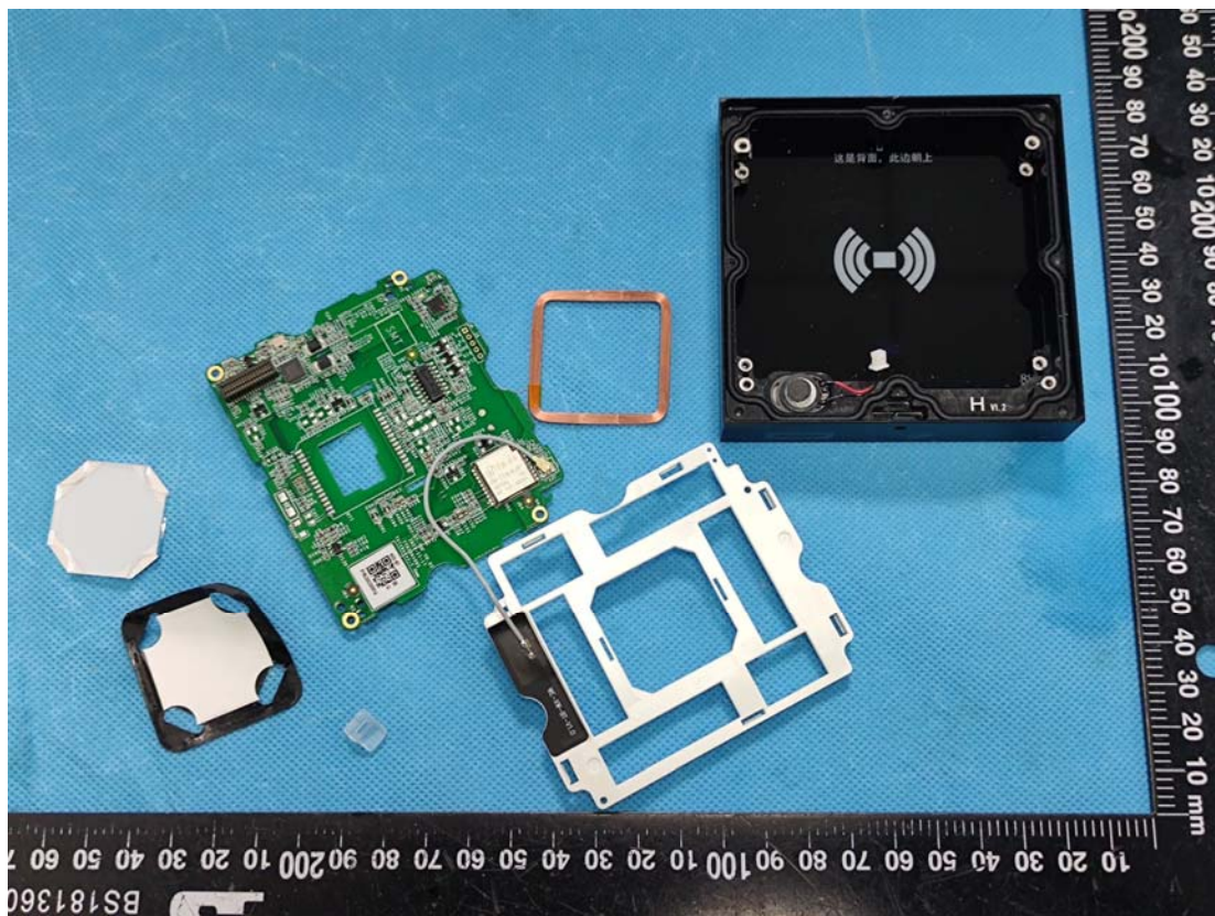
BLE Antenna
