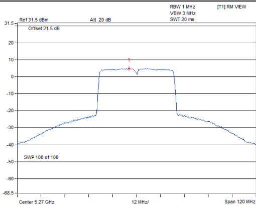
802.11ax (HE40)_Chain 0 / CH54
