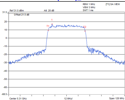
802.11ax (HE40)_Chain 0 / CH62
