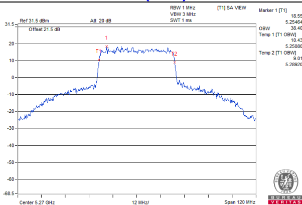
802.11ax (HE40) / CH54
