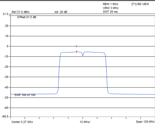
802.11ax (HE40)_Chain 0 / CH54
