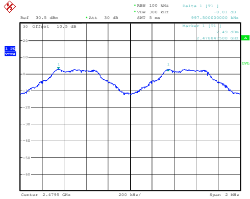
DH1_High 0.998MHz
