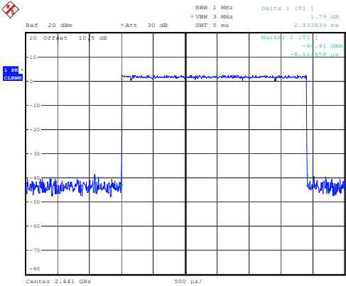
\pi/4 -DQPSK_Hopping_2DH5 2.934ms
