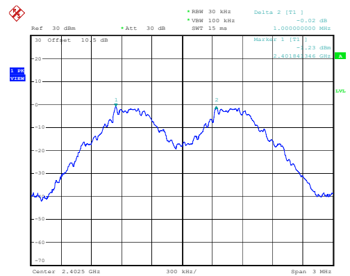
GFSK_Low 1.000MHz
