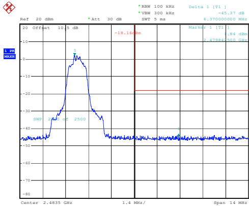
\pi/4 -DQPSK_High
