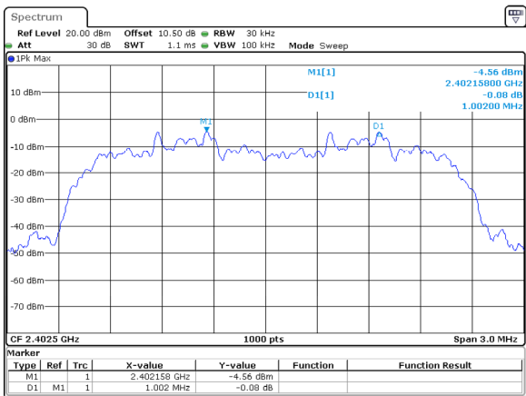
\pi/4 -DQPSK_Low 1.002MHz
