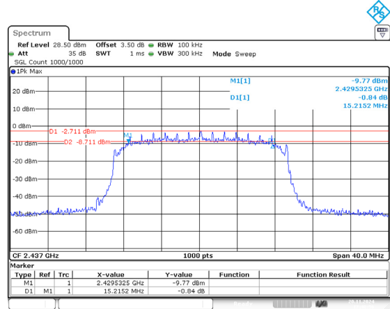
802.11n20_2437MHz 15.215MHz
