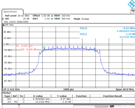
802.11n20_2412MHz 15.215MHz
