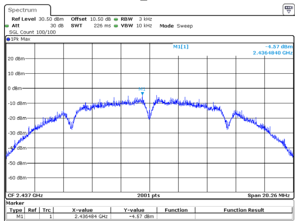
802.11b_2437MHz
