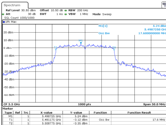
802.11n20_5500MHz
