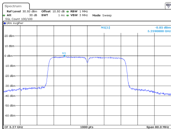
802.11n40_5270MHz
