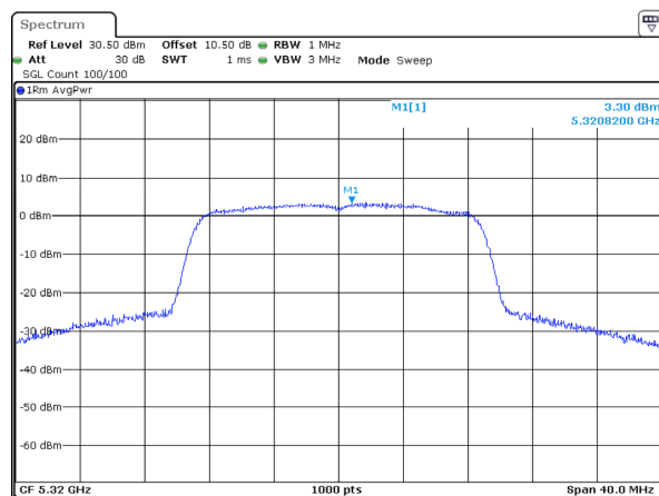
802.11n20_5320MHz
