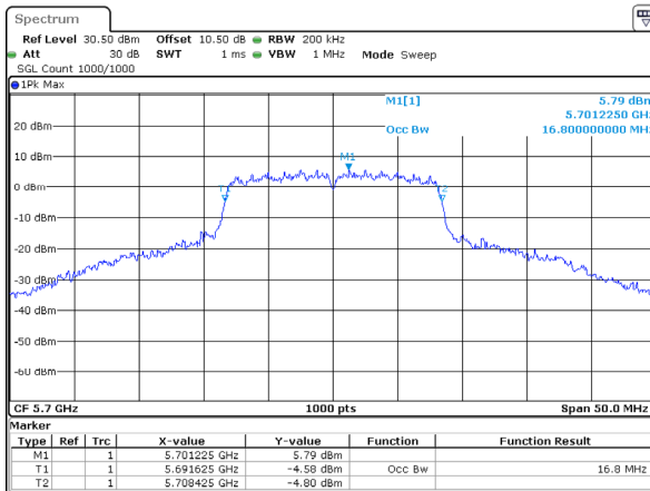
802.11a_5700MHz
