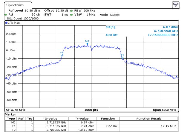
802.11a_5720MHz
