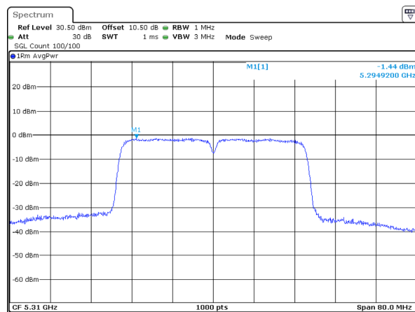
802.11n40_5310MHz
