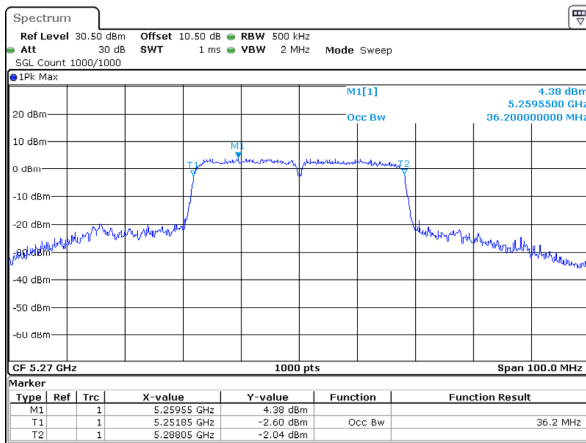
802.11n40_5270MHz
