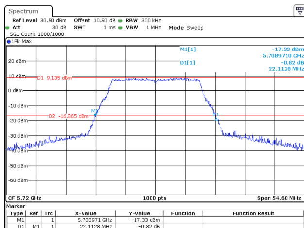
802.11a_5720MHz
