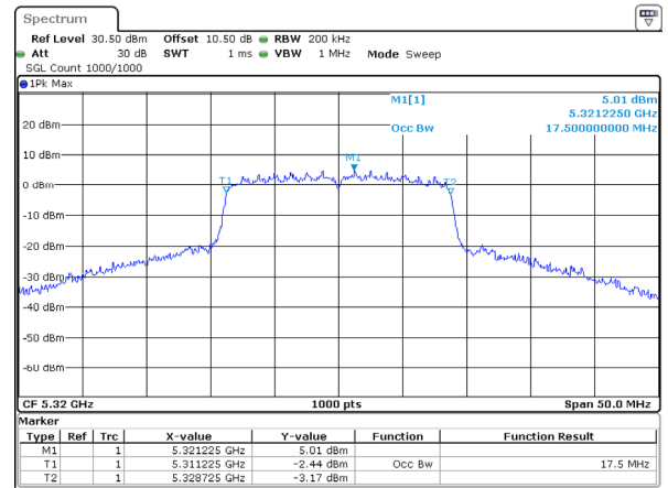
802.11n20_5320MHz
