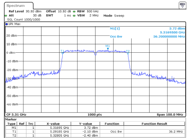
802.11n40_5310MHz
