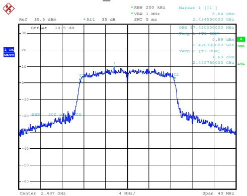
802.11n20_2437MHz 17.450MHz
