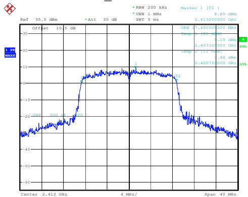
802.11n20_2412MHz 17.450MHz
