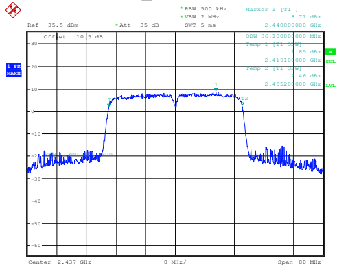
802.11n40_2437MHz 36.100MHz
