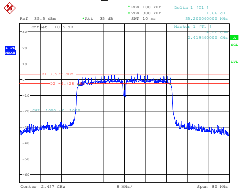
802.11n40_2437MHz 35.200MHz
