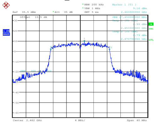
802.11n20_2462MHz 17.450MHz
