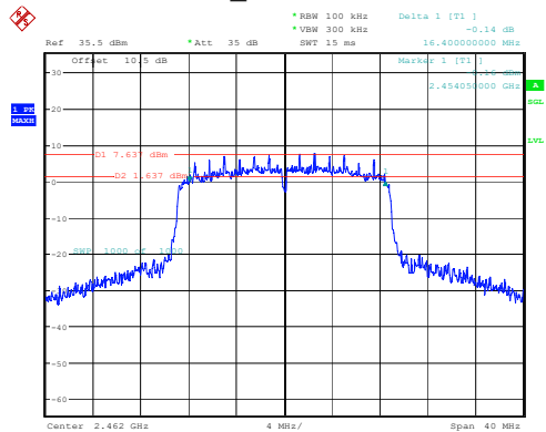
802.11n20_2462MHz 16.400MHz
