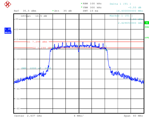
802.11n20_2437MHz 16.400MHz
