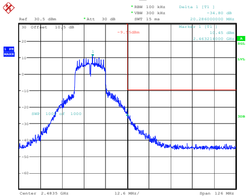
802.11n20_2462MHz
