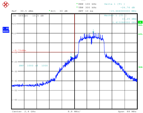
802.11n20_2412MHz
