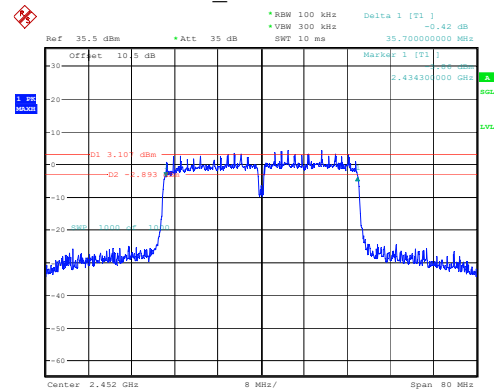
802.11n40_2452MHz 35.700MHz
