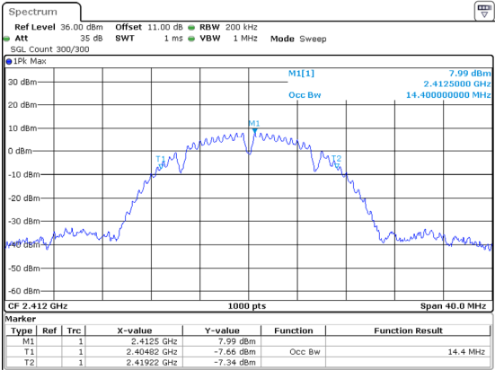
802.11b_2412MHz
