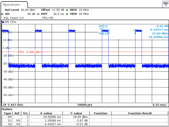
802.11n20_2437MHz
