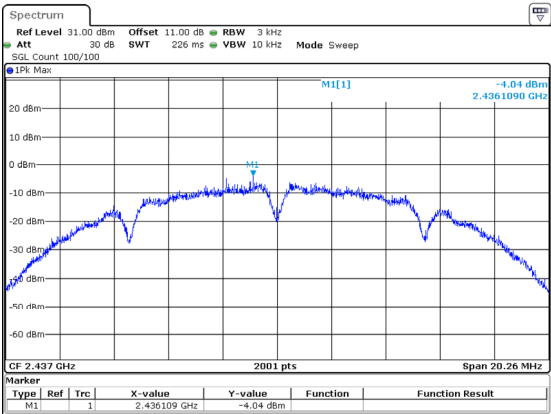
802.11b_2437MHz
