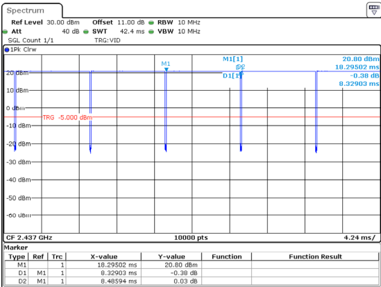
802.11b_2437MHz
