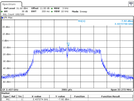
802.11g_2437MHz
