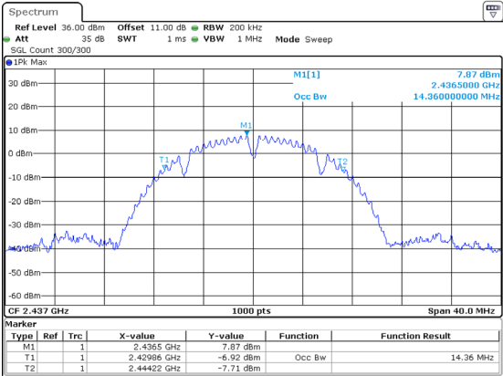
802.11b_2437MHz
