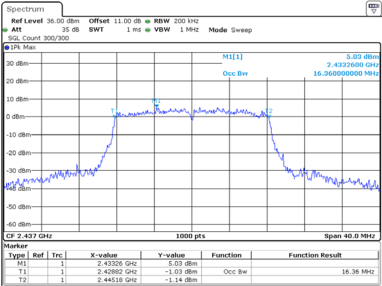
802.11g_2437MHz
