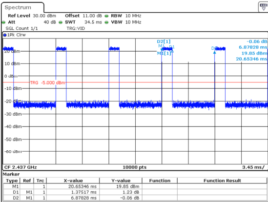
802.11g_2437MHz
