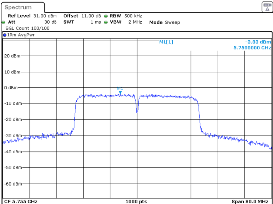
802.11n40_5755MHz
