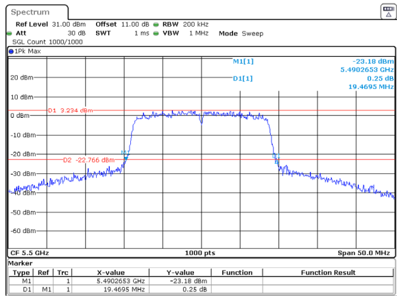
802.11n20_5500MHz
