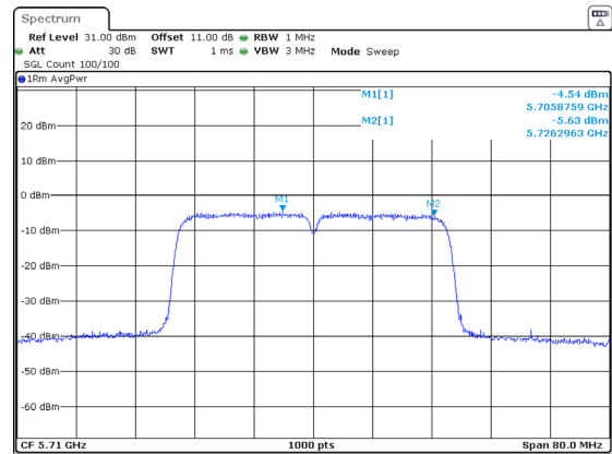
802.11n40_5710MHz
