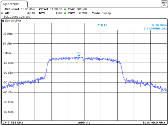
802.11n20_5785MHz
