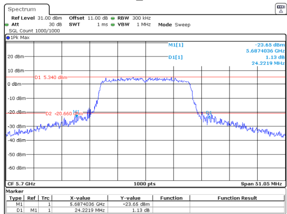
802.11a_5700MHz
