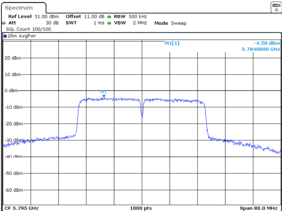
802.11n40_5795MHz
