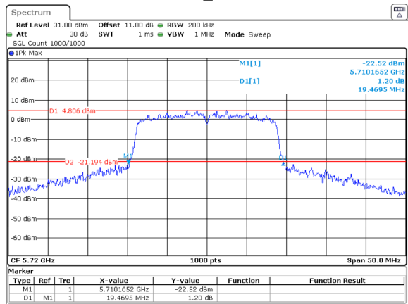
802.11n20_5720MHz
