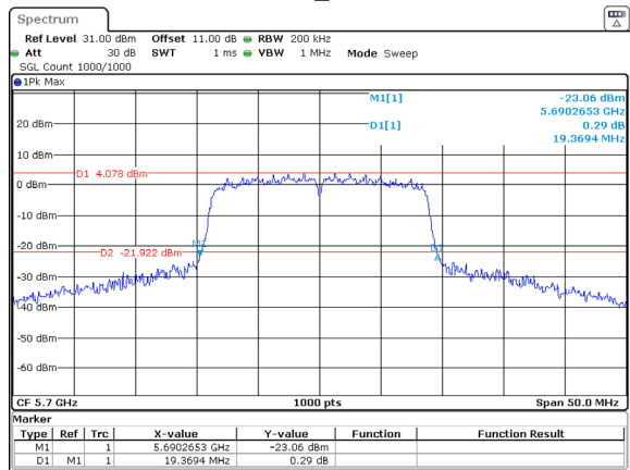
802.11n20_5700MHz
