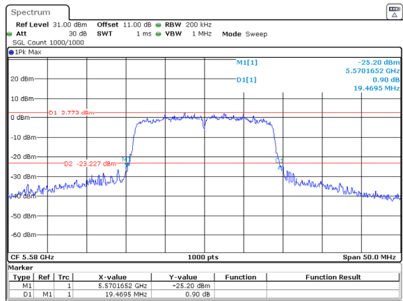
802.11n20_5580MHz
