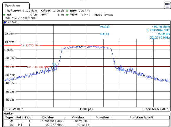
802.11a_5720MHz
