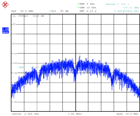
802.11b_2462MHz
