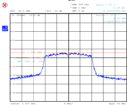
802.11g_2437MHz
