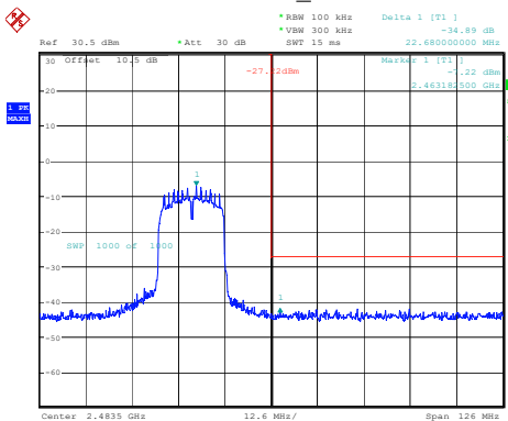
802.11n20_2462MHz
