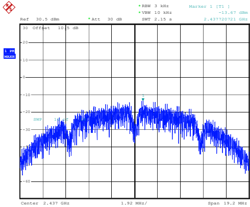
802.11b_2437MHz
