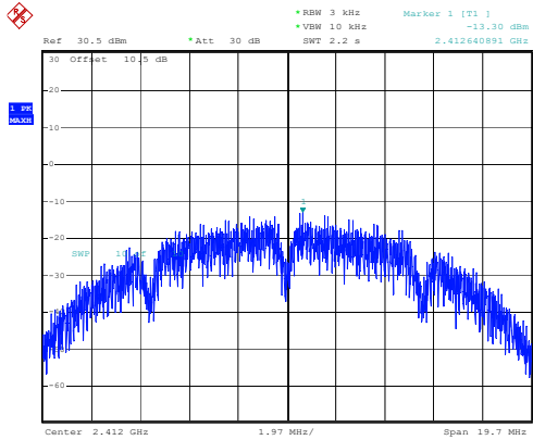
802.11b_2412MHz
