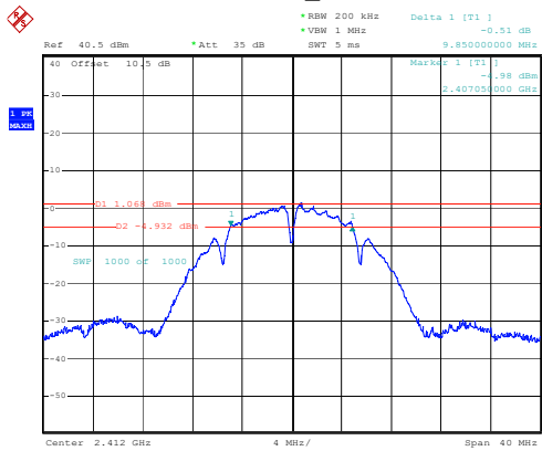
802.11b_2412MHz
