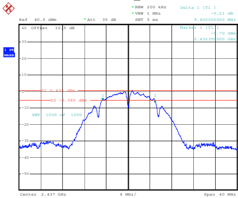
802.11b_2437MHz
