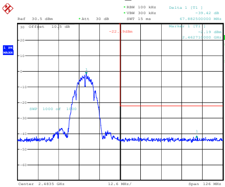
802.11b_2462MHz
