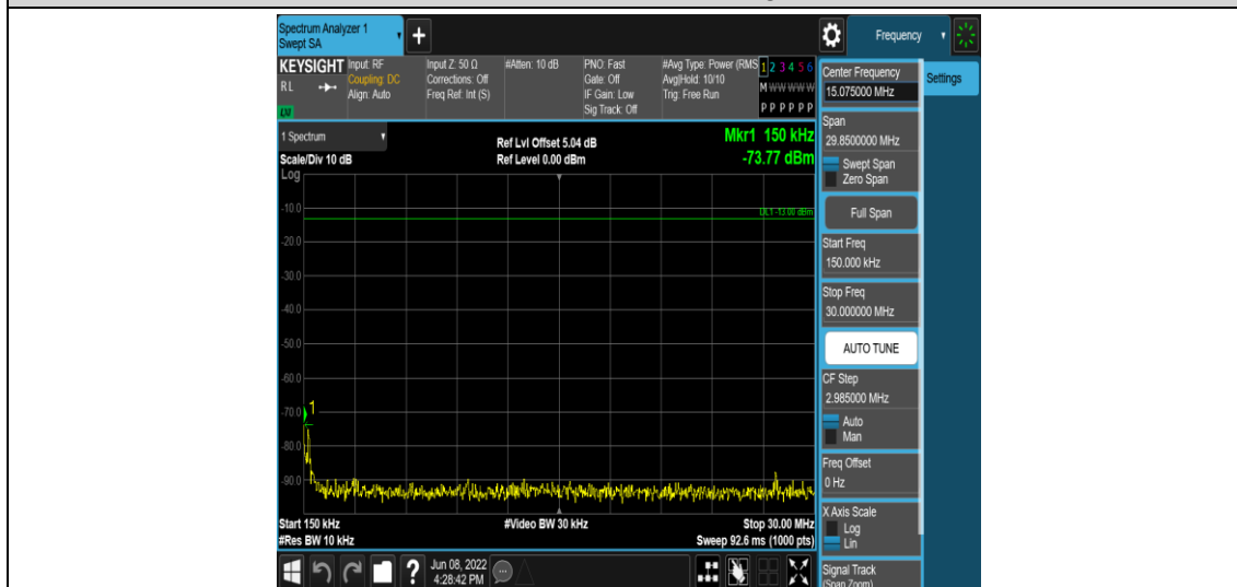
Band41-5MHz-QPSK-40740-1RB#0-Range2:0.15~30MHz
