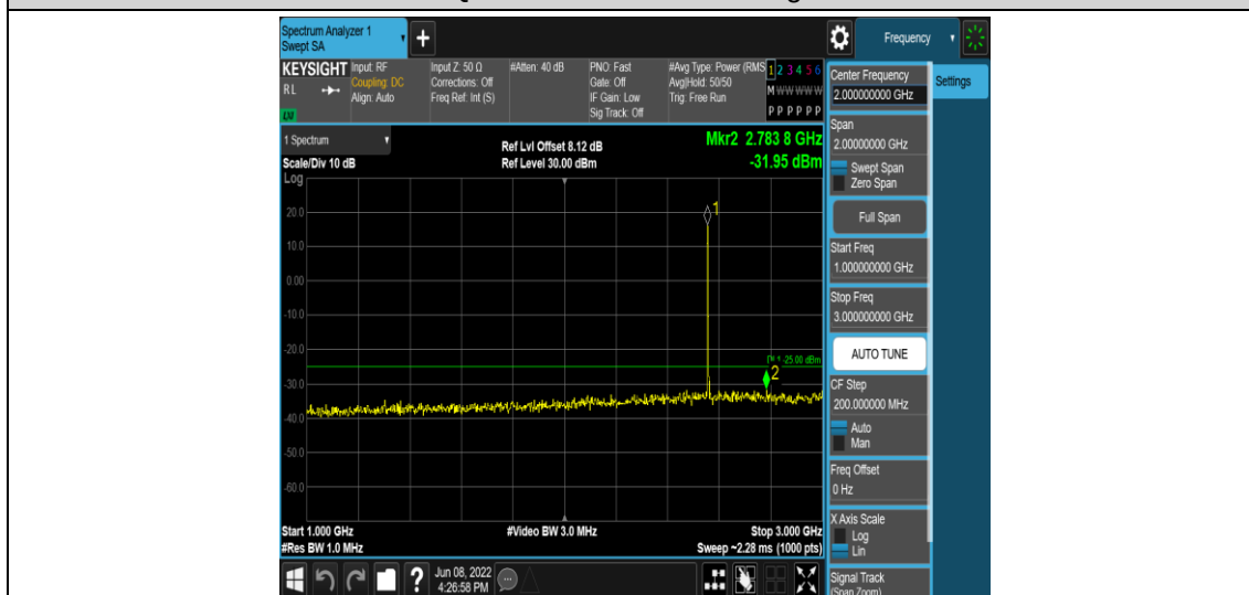
Band41-5MHz-QPSK-40265-1RB#0-Range4:1000~3000MHz
