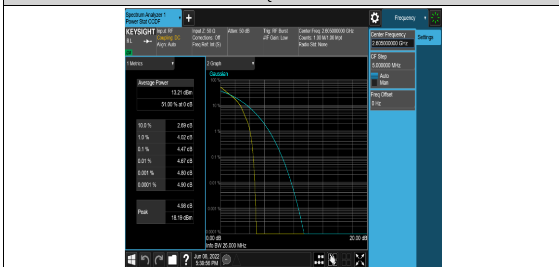
Band41-20MHz-QPSK-40740-1RB#0
