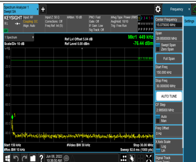
Band40-5MHz-QPSK-38750-1RB#0-Range2:0.15~30MHz
