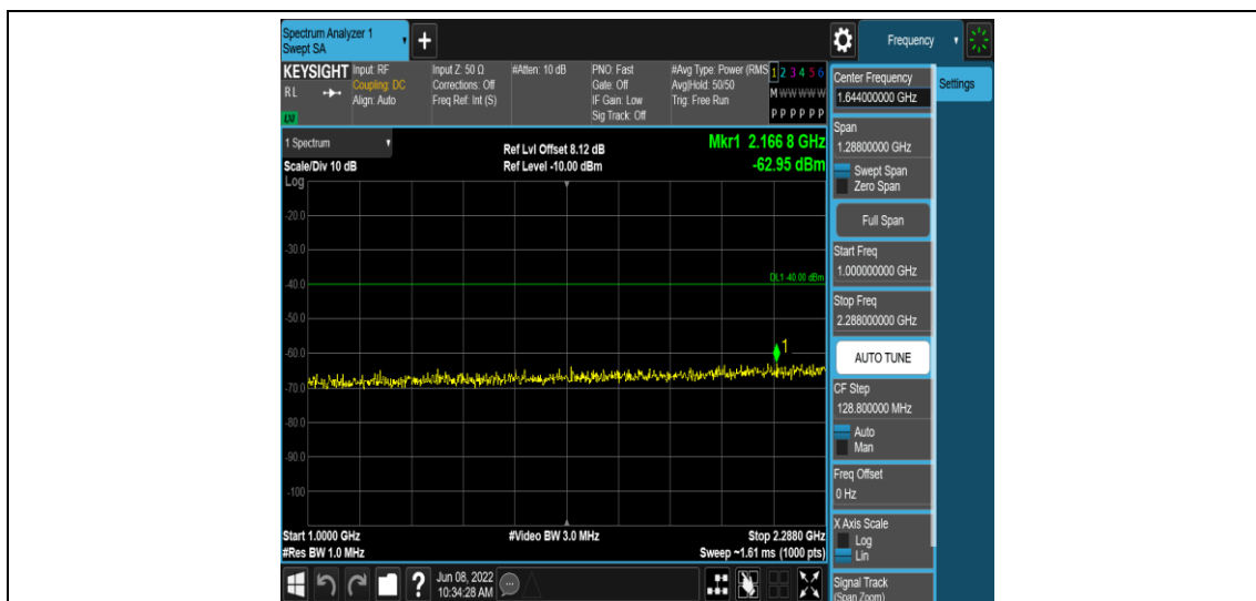
Band40-5MHz-16QAM-38725-1RB#0-Range4:1000~2288MHz
