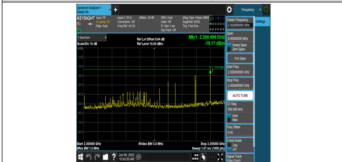
Band40-5MHz-QPSK-38775-1RB#0-Range8:2300~2305MHz
