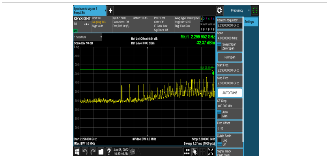
Band40-5MHz-QPSK-38750-1RB#0-Range7:2296~2300MHz
