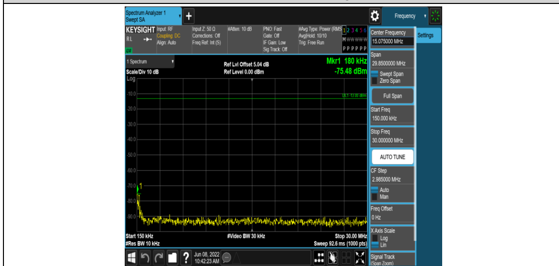
Band40-5MHz-QPSK-38775-1RB#0-Range2:0.15~30MHz
