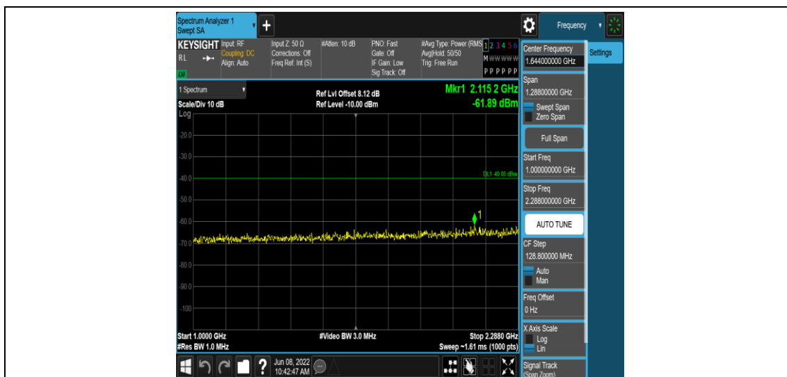
Band40-5MHz-QPSK-38775-1RB#0-Range4:1000~2288MHz
