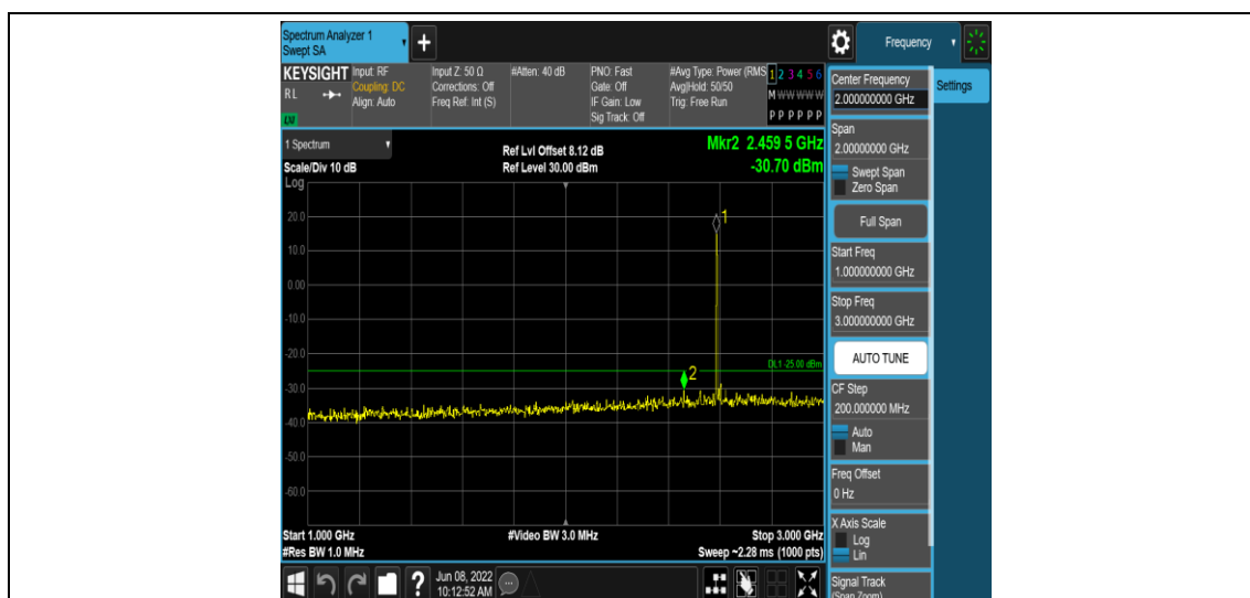
Band38-20MHz-QPSK-38000-1RB#0-Range4:1000~3000MHz
