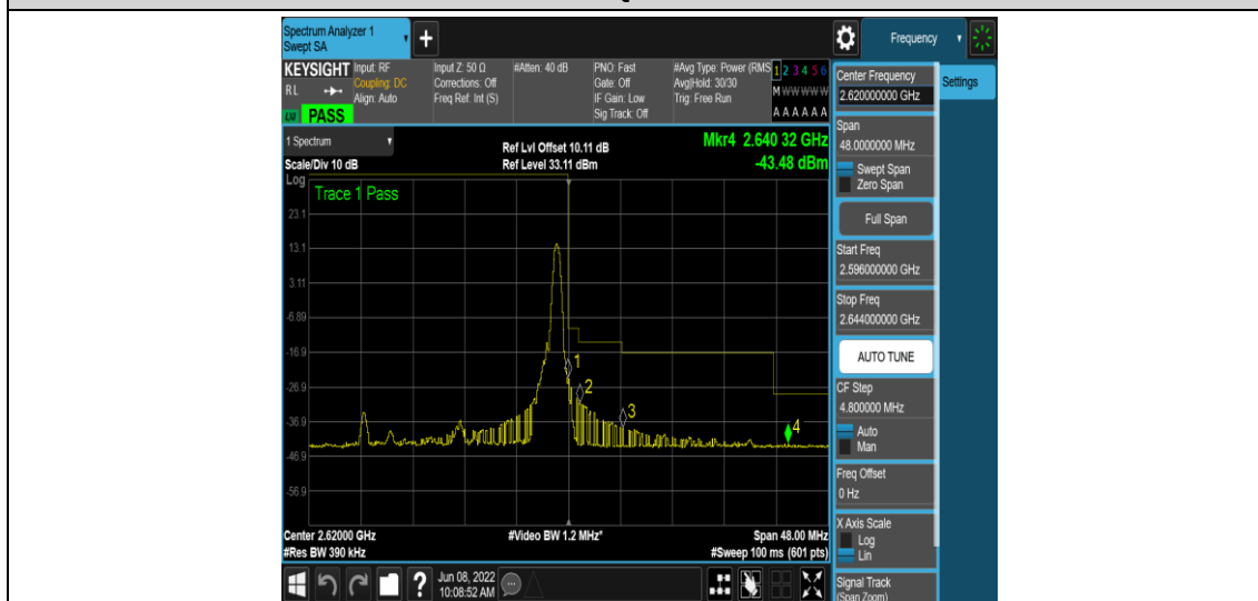
Band38-20MHz-QPSK-38150-1RB#99
